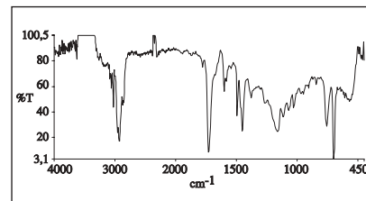
Infrardeči spekter tonerja za laserski tiskalnik Hewlett Packard HP Laserjet
